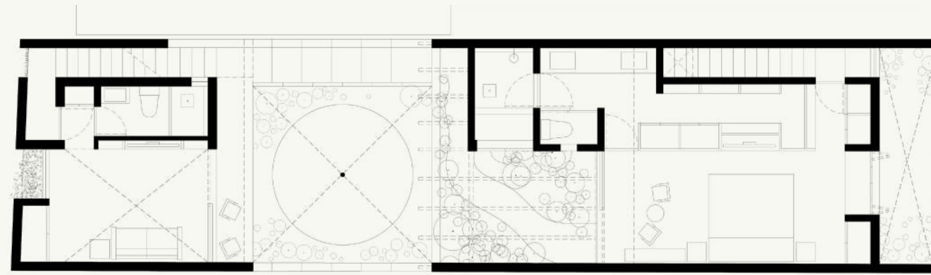
Planta Alta
